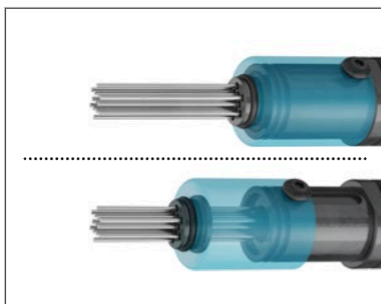
Verstellbarer Nadelschlitten mit integrierter Nadelführung gewährleistet lange Standzeiten
